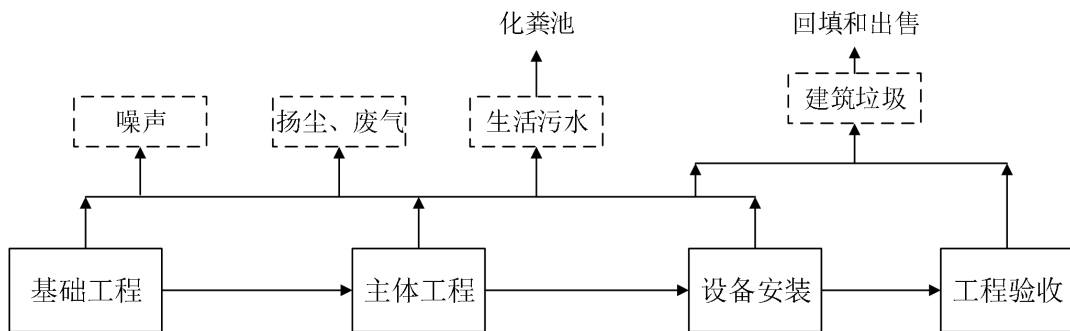
图1 施工期工艺流程图
