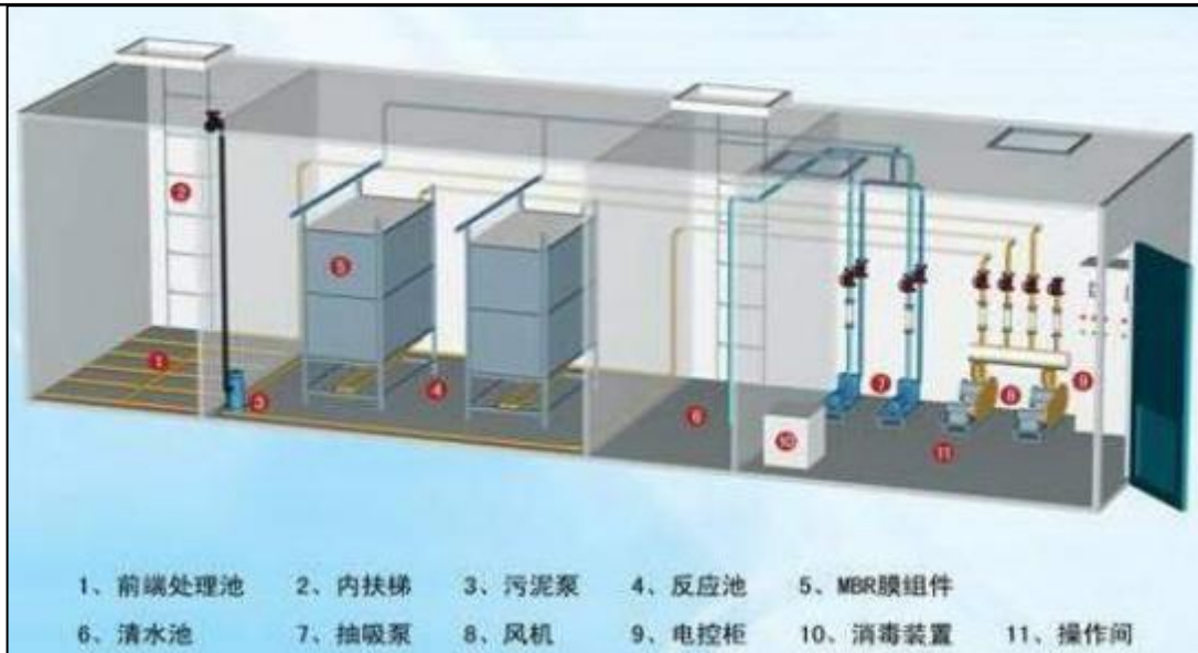
图3 MBR 污水处理系统构造图
