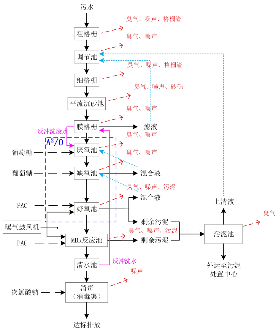
图 2 项目污水处理设施工艺流程图
