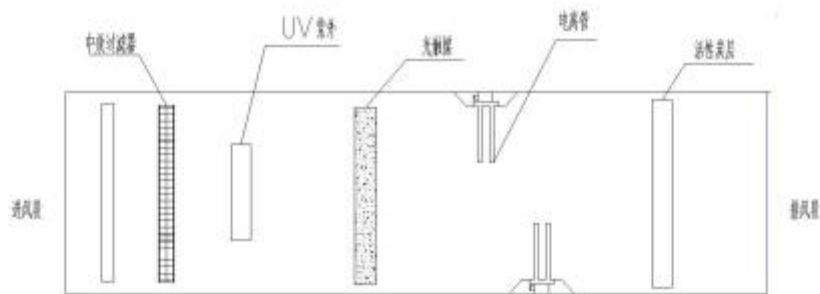
图 8 离子除臭装置示意图
